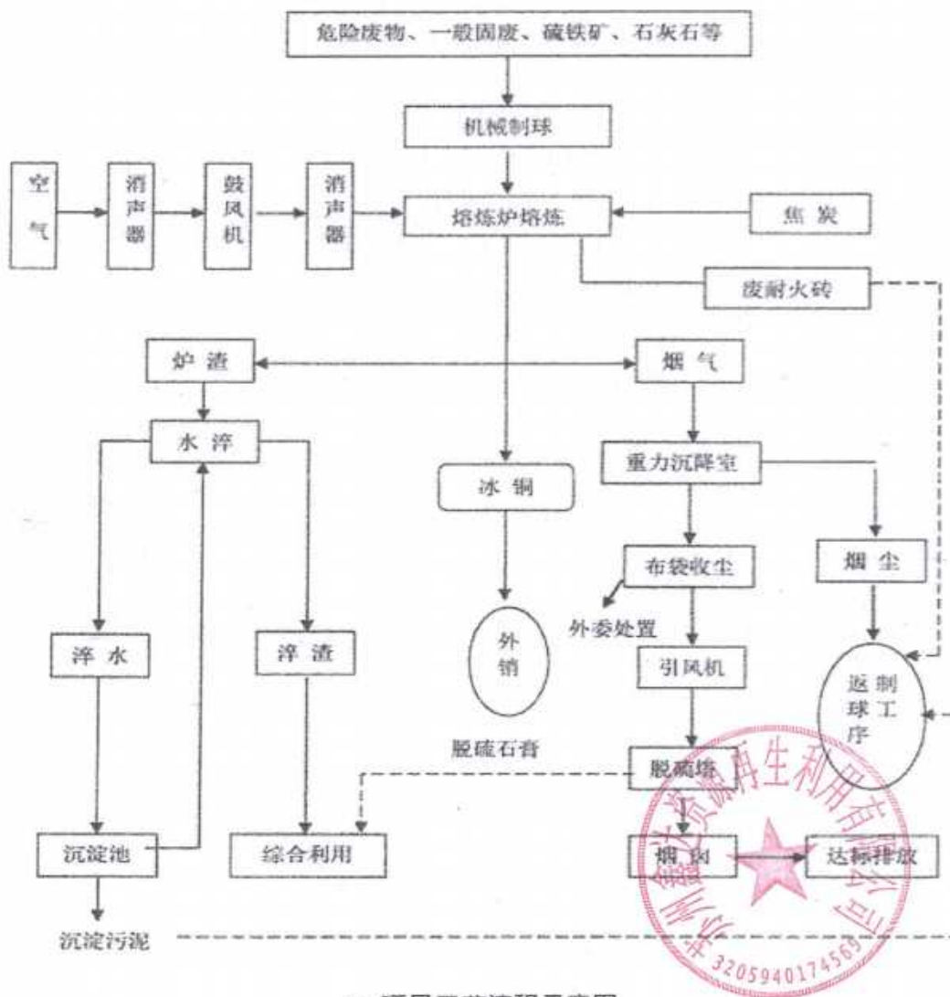
1-1 项目工艺流程示意图
